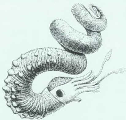
Reconstructie van een Didymoceras nebrascense . - Ammonites and other Cephalopods of the Pierre Seaway: Identification Guide : 49.
